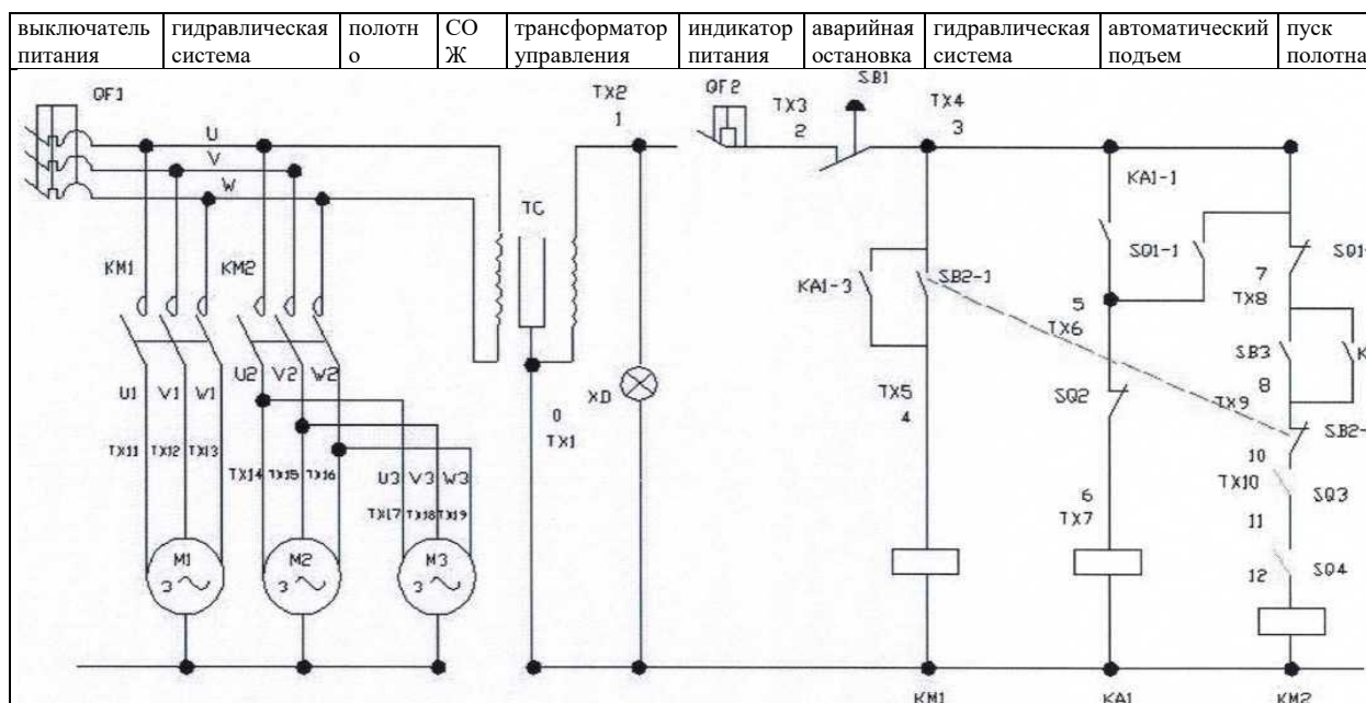
Рисунок 7. Принципиальная электрическая схема ленточнопильного станка Metal Master MSK-350
