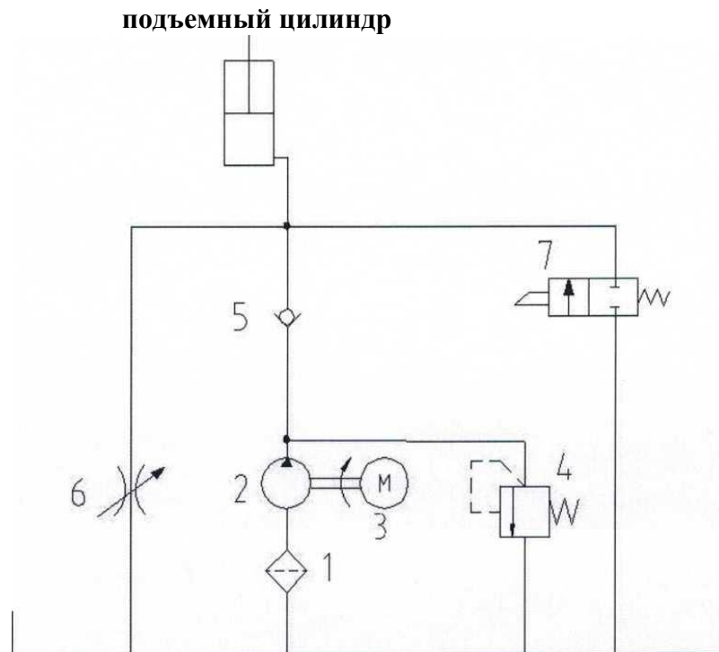
Рисунок 6. Схема гидравлической системы ленточнопильного станка Metal Master MSK-350
