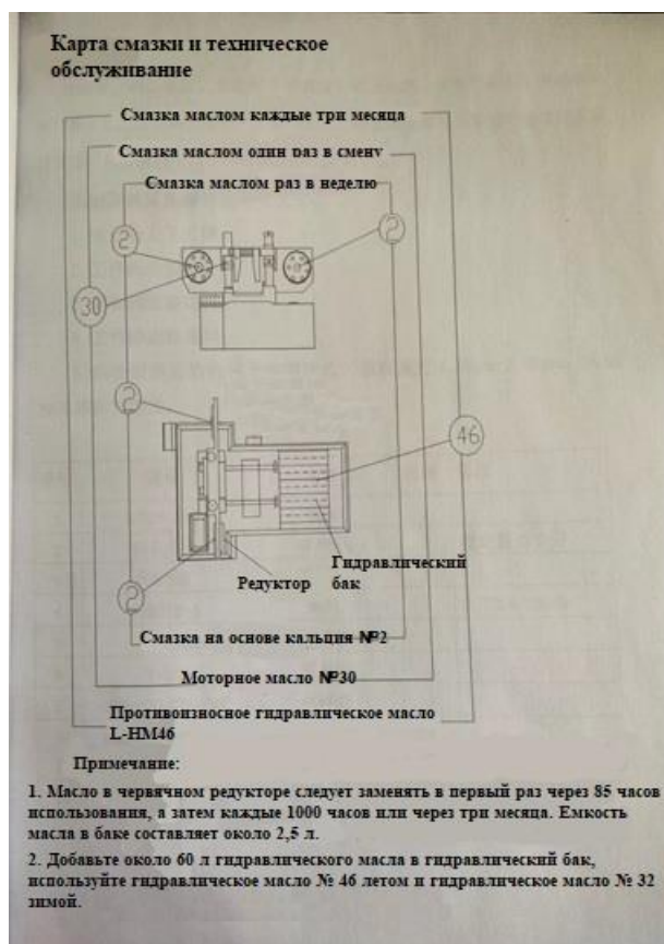
Рисунок 8. Карта смазки и техническое обслуживание ленточнопильного станка Metal Master MSK-350
